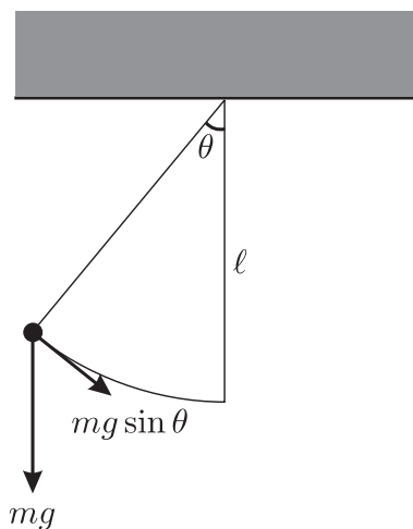
圖3. 單擺運動
